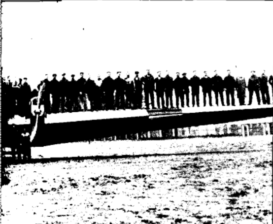
Un Junker G-23, se le sometió a la respetable prueba de hacer soportar a sus alas el peso de sesenta toneladas a lo largo del aparato.
