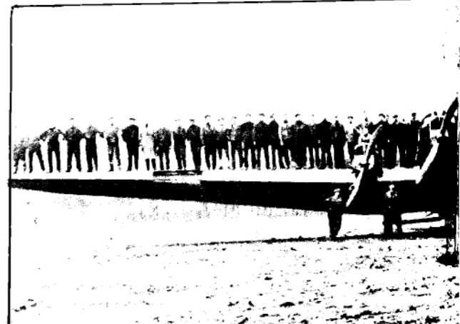
Para probar la resistencia del nuevo aeroplano gigante al prueba que puede apreciarse en esta fotografía, consistentemente en hombres colocados en fila a toda
